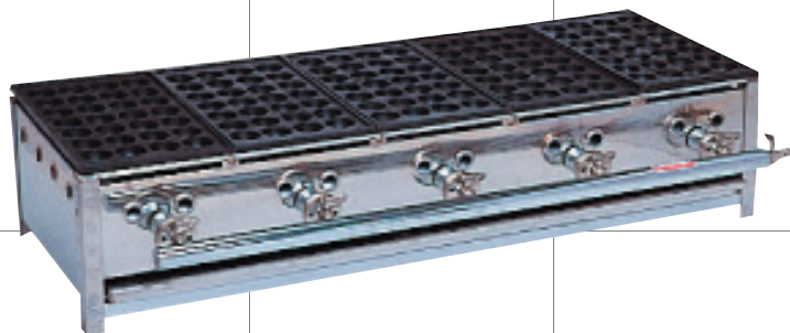
■小型たこ焼き機 84個 W560×D350×H230mm ■たこ焼き機 140個 W970×D340×H230mm
